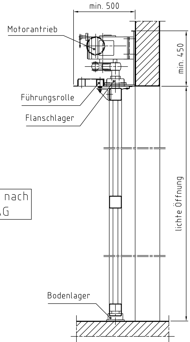
Schnitt B-B
